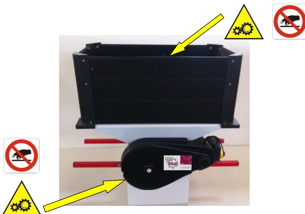
Fig. 2 Elemente mobile în mișcare
